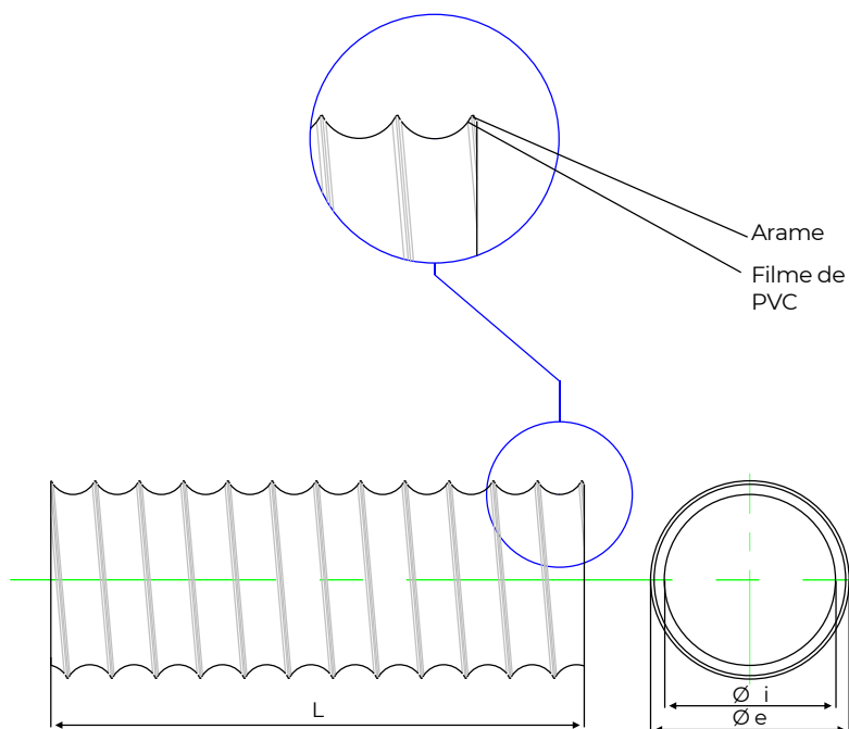
Desenho Técnico
