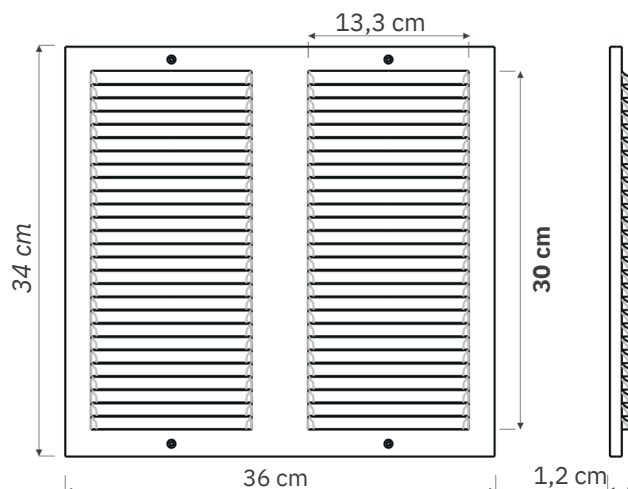
Desenho Técnico
