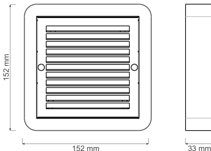
Desenho Técnico
