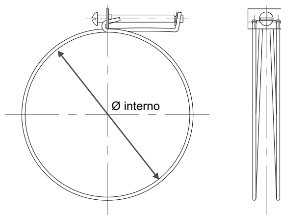
Desenho Técnico
