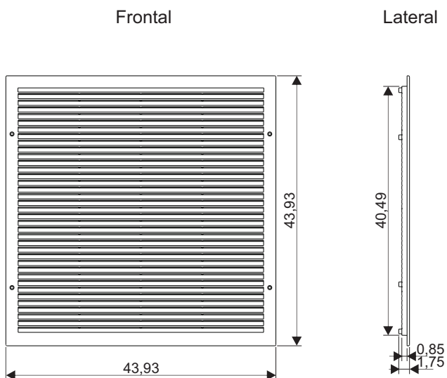
Desenho Técnico
