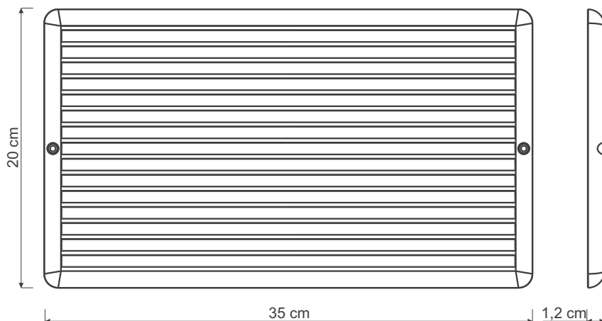
Desenho Técnico
