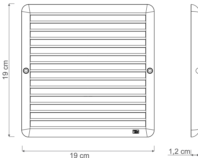
Desenho Técnico
