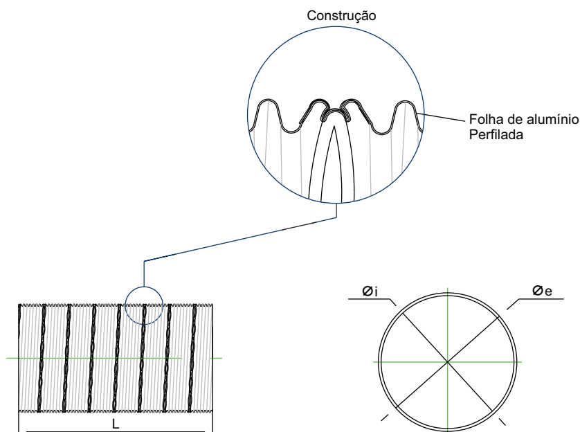
Desenho Técnico
