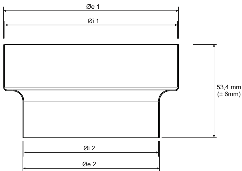
Desenho Técnico
